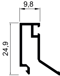
G-115 Isıcam Çıta 0,231 kg/m
