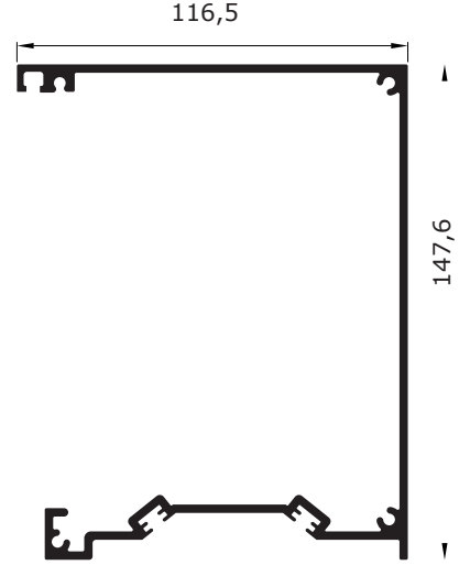
SP-101 Şase 3,335 kg/m
