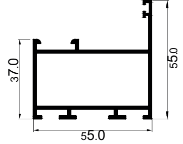
KK-1020 Kanat 1,000 kg/m
