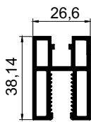
G-127 Tekcam Geniş Dkey Baza 0,832 kg/m
