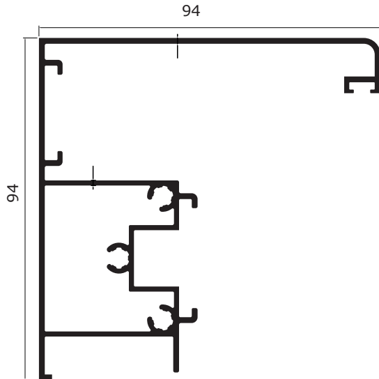
RK-107 Rüzgar Kırıcı Dikme(Motorlu) 1,750 kg/m
