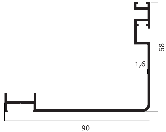
RK-108 Rüzgar Kırıcı Dikme Kapak(Motorlu) 0,900 kg/m
