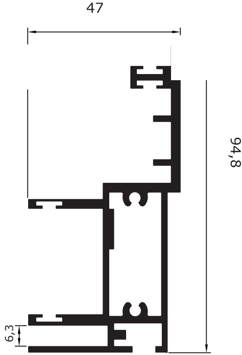
RK-103 Sabit Dikme 2.210 kg/m
