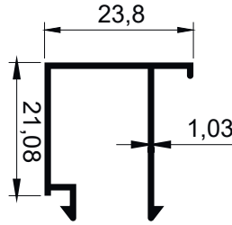
G-116 Tek Cam Çıta 0,292 kg/m
