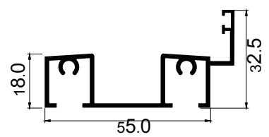
KK-1080 Eşikli Alt Kasa 0,750 kg/m
