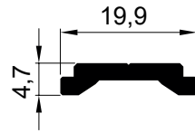
G-114 Vasistas kanat tij 0,155 kg/m
