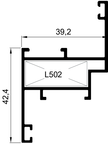
G-112 Vasistas kanat 0,708 kg/m
