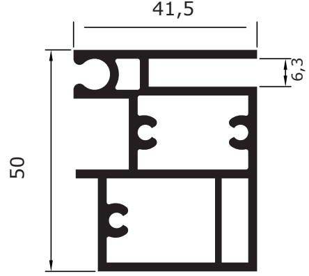
RK-102 Hareketli Dikme/Yatay 1.580 kg/m
