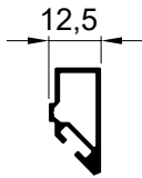
G-113 Vasistas Kanat Adaptör 0,277 kg/m
