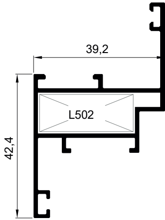
G-112 Vasstas Kanat 0,708 kg/m
