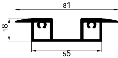
KK-1040 Eşiksiz Alt Kasa 1,050 kg/m
