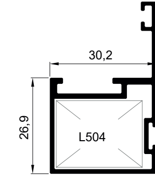
G-111 Kalın Vasstas Kasa 0,970 kg/m
