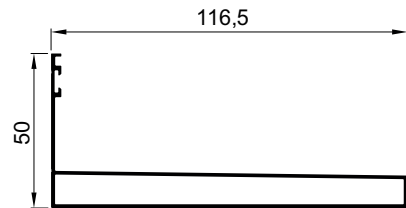
G-117 Isıcam Alt Kasa 0,973 kg/m
