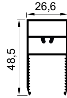
G-105 Sabit Kanat Yatay Alt Baza 0,690 kg/m
