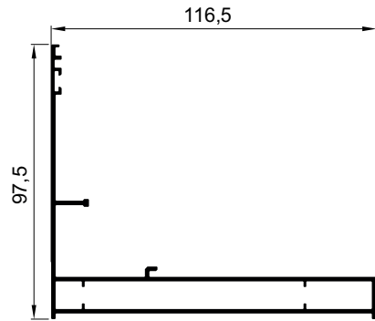
G-107 Isıcam Yan Kasa 1,613 kg/m
