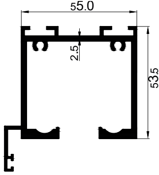
KK-1010 Üst Kasa 1,750 kg/m
