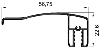
G-128 Tekcam Geniş Küpeşte 1,472 kg/m
