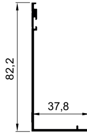
G-109 Isıcam Yan Kasa Dış Kapak 0,565 kg/m
