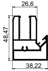
G-129 Tekcam Kalın Seri Çekme Baza 1,220 kg/m
