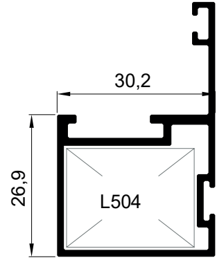
G-111 Kalın Vasistas Kanat 0,970 kg/m
