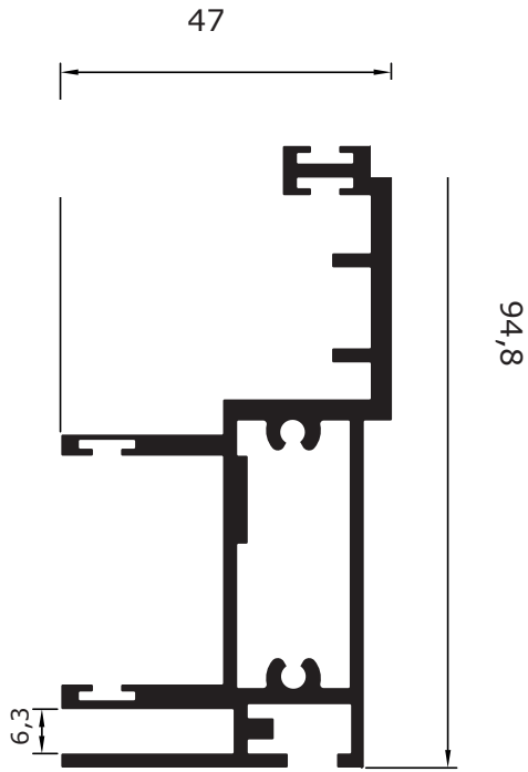
RK-103 Sabit Dikme 2.210 kg/m
